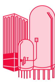
L'oxygène liquide
